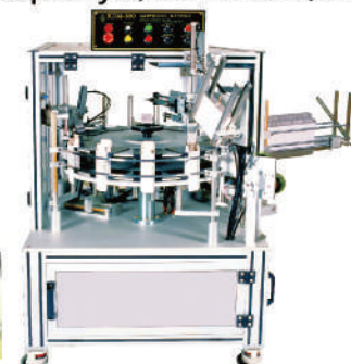
裝盒機
