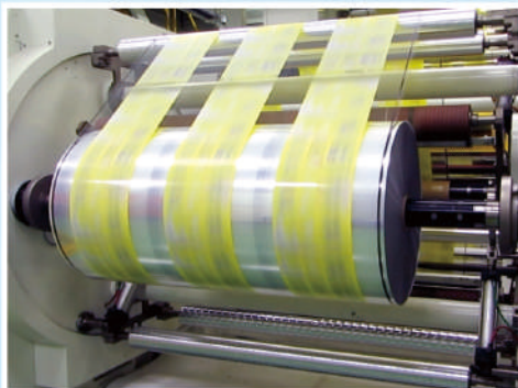
塑料包材 - 八色水性柔版印刷設備
