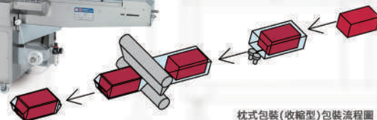
全自動枕式包裝生產線
