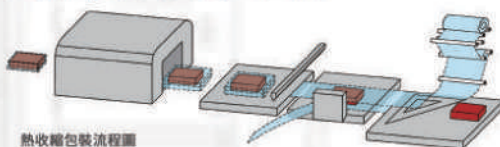
熱收縮包裝流程圖
